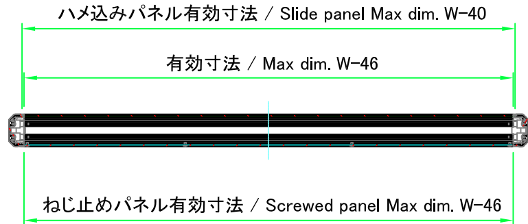
A-A ( 1 : 8 )
