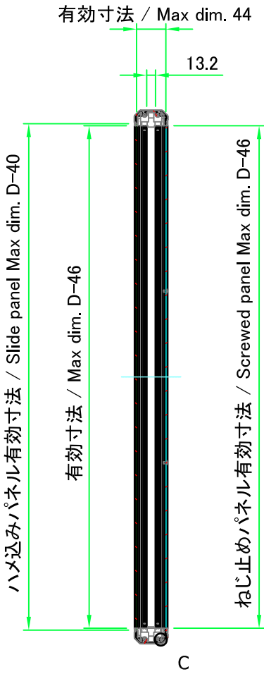
B-B ( 1 : 8 )
